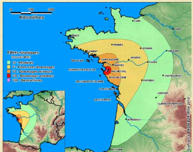
Isoséismes du séisme du marais Breton du 25 janvier 1799, à partir des données SisFrance
